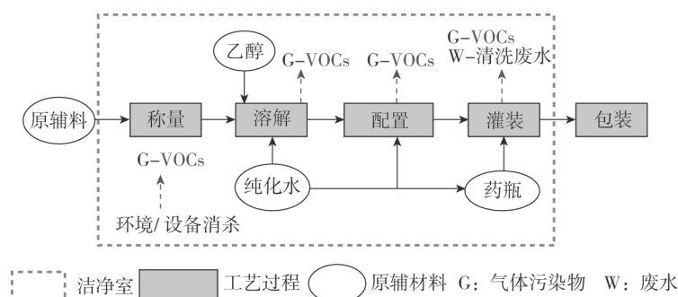
图 2-4 气体制剂生产工艺流程及产排污节点
