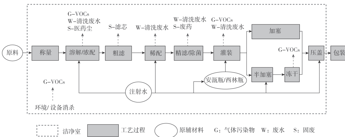
图 2-2 液体制剂工艺流程及产排污节点
