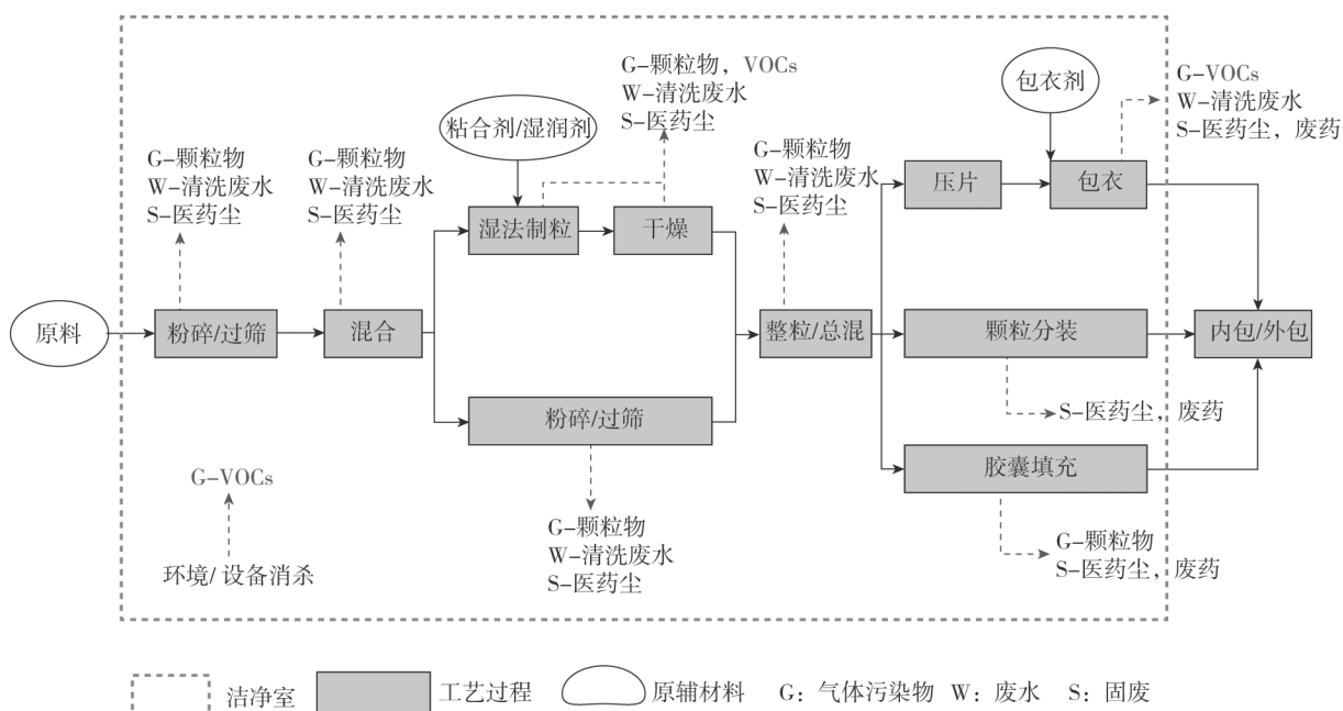
图 2-1 固体制剂工艺流程及产排污节点
