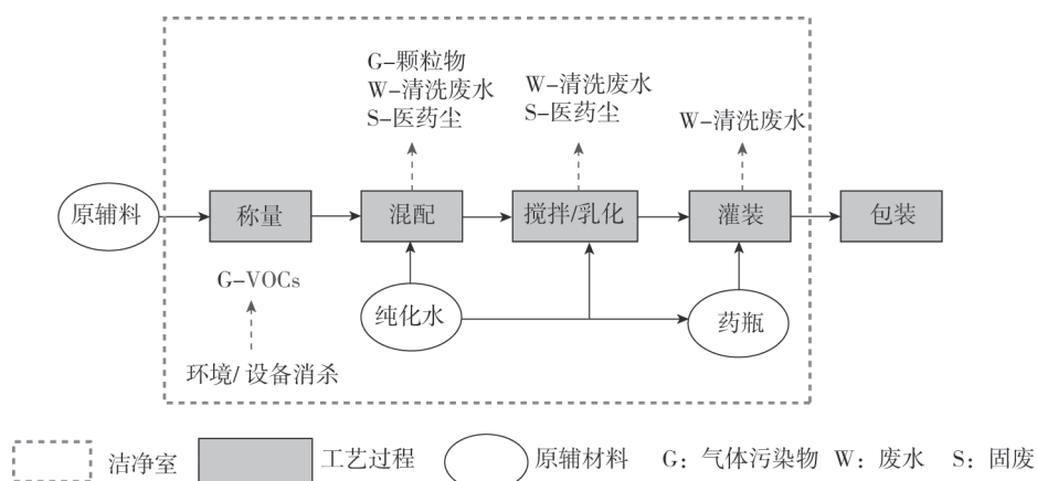
图 2-3 半固体制剂生产工艺流程及产排污节点
