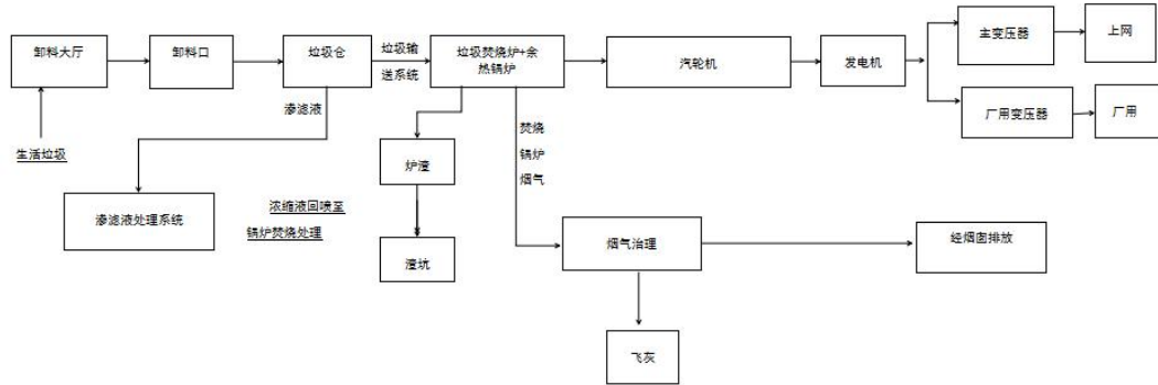
图 2-1 生活垃圾焚烧发电工艺流程图
