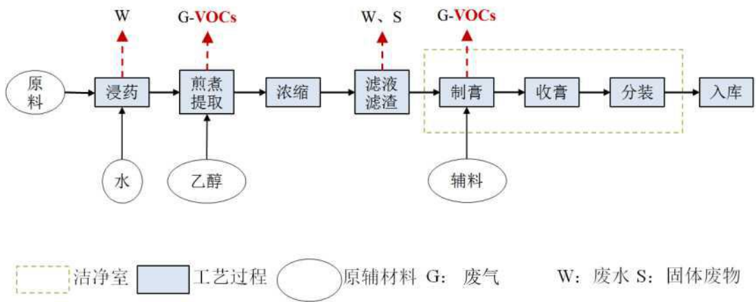
图 2-3 半固体制剂生产工艺流程及排污节点
