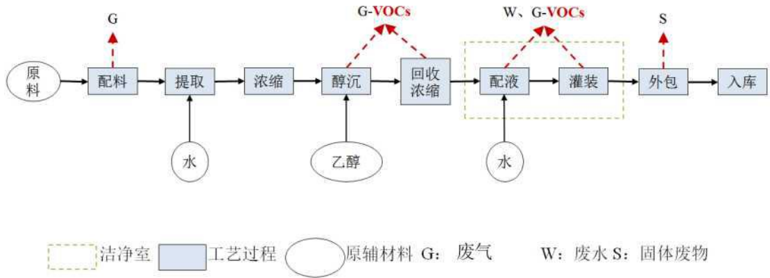
图 2-2 液体制剂工艺流程及排污节点
