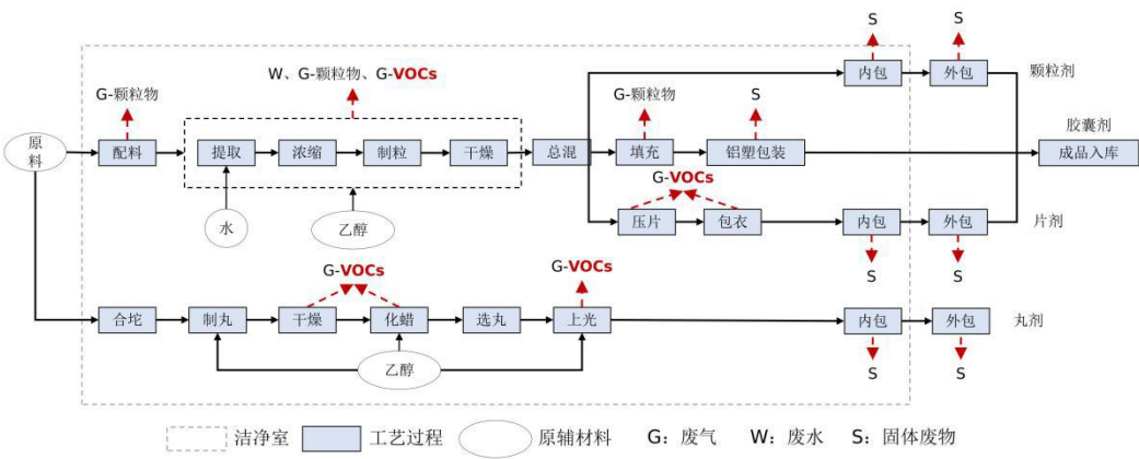
图 2-1 固体制剂的工艺流程及排污节点
