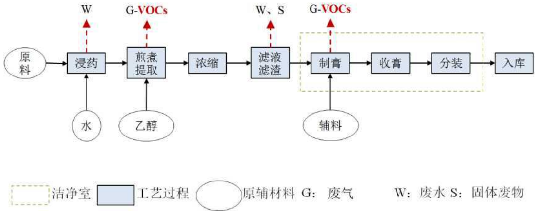
图 2-3 半固体制剂生产工艺流程及排污节点
