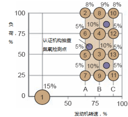
图 3.1 ESC 测试循环
